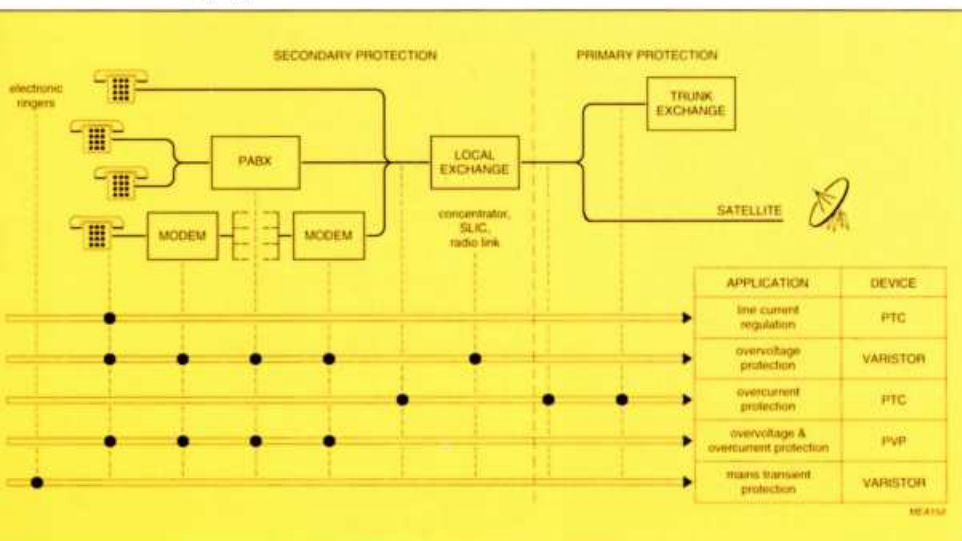
Afb. 1. Blokschema van een telefoonstelsel, waarin de plaatsen zijn aangegeven waar PTC-thermistors en varistors kunnen worden gebruikt voor zowel primaire als secundaire beveiliging.
